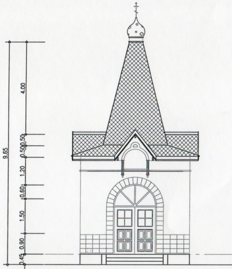
① 4.50 ② รูปด้าน 1
